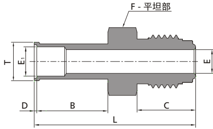
"H" 型自动卡套管焊接接头
